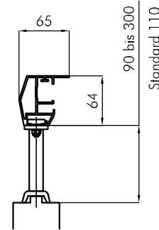
Führungsschiene mit Distanzkonsole U-XL guiding rail with distance bracket U-XL
