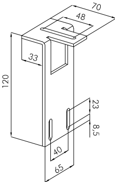
Winkel für Stegmontage DFS support for bar assembly DFS
