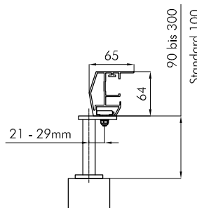
Halter Führungsschiene XL einseitig Support for single guiding rail
