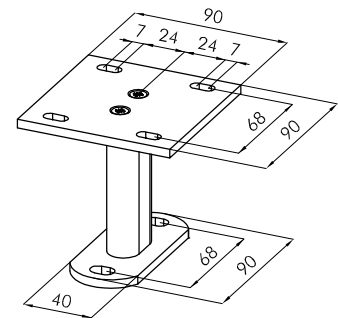
Halter Führungsschiene zweiseitig Support for double guiding rail
