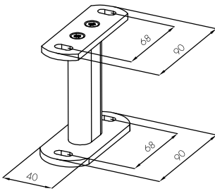
Distanzkonsole XL distance bracket XL
