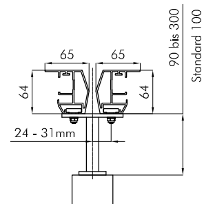
Halter Führungsschiene zweiseitig Support for double guiding rail
