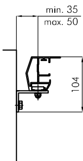
Führungsschiene mit Laibungswinkel guiding rail with support for reveal mounting
