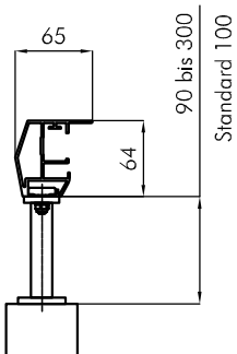
Führungsschiene mit Distanzkonsole guiding rail with distance bracket
