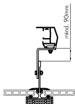
Führungsschiene mit Falzmontage guiding rail with bar assembly
