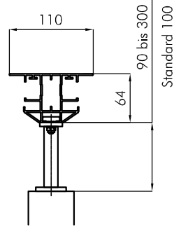
Mittenführungsschiene mit Distanzkonsole centre guiding rail with distance bracket
