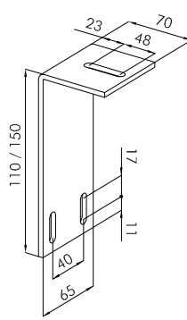
Winkel für Stegmontage SFS support for bar assembly SFS
