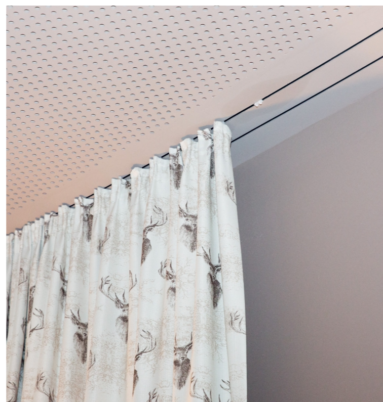
Nosný profil TP-FLEX dvoudrážkový s plastovými drážkami pro uchycení závěsu
