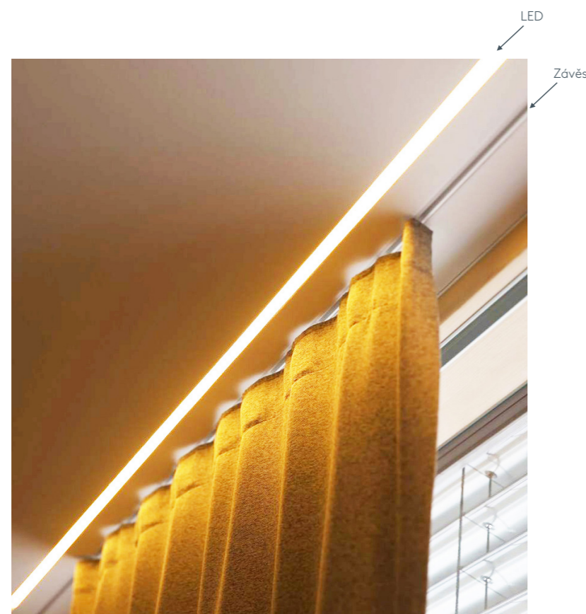
Nosný profil TP-FLEX dvoudrážkový s LED světelným profilem a drážkou pro uchycení závěsu (LED na místě: Doporučení min. 120 LED světelných bodů na bm)
