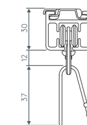
Rolery 5028 s kovovým háčkem 4806
